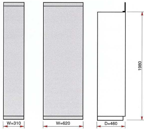
Colonnes Type LSF simples ou doubles
